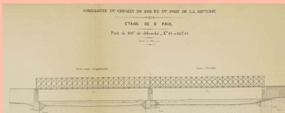
Plan de la Cie du Chemin de fer et du Port de la Réunion - Pont ferroviaire – 100 m de débouché – de l'Étang de Saint Paul (archives départementales)
